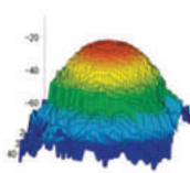
US-103S (3MHz) BFA: 0.8um \pm 20% (IEC) + 0.8um \pm 20% (FDA) BFR: 2.4 \pm 30% (IEC) + 3.4 \pm 30% (FDA)
